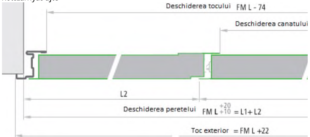
Kétszárnyas ajtó
