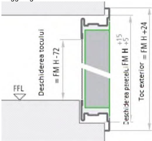
Ajtó belső és külső küszöbvel Függőleges rész
